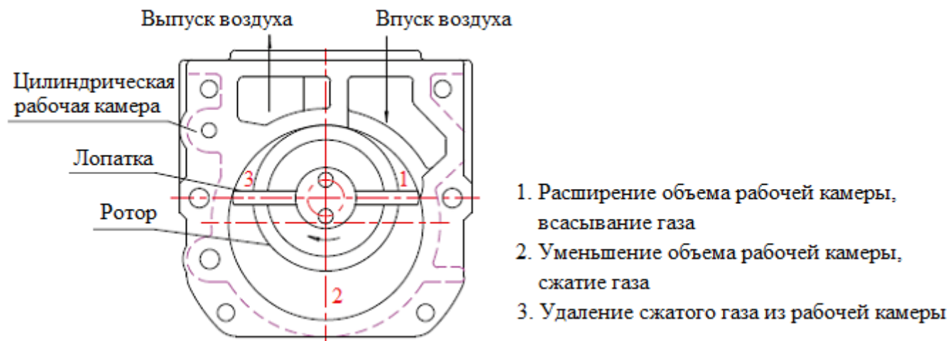
Рис. 2 – Внешний вид насоса VRD
