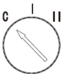
Рис. 6 – Клапан газобалласта насосов серии VRD
