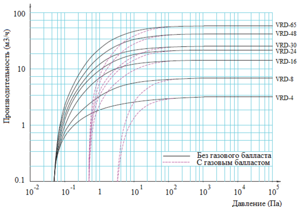
Рис. 3 – Зависимость производительности от давления
