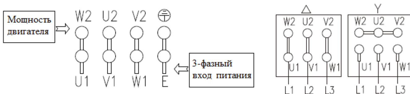
Рис. 4 – Схема подключения 3 проводов (слева) и 6 проводов (справа) трехфазного электродвигателя насосов серии VRD
